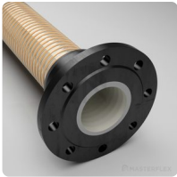
Flangia fissa Combiflex in PU, montata in modo permanente Flangia in PU integrata per tutti i tubi Master-PUR, per controflange secondo DIN 2632 / DIN 2633 / DIN 2673
