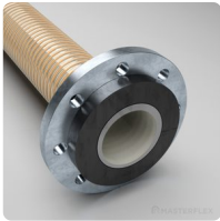
Flangia mobile Combiflex in PU, montata in modo fisso Flangia fusa in PU per tutti i tubi Master-PUR, per controflange secondo DIN 2632 / DIN 2633 / DIN 2673
